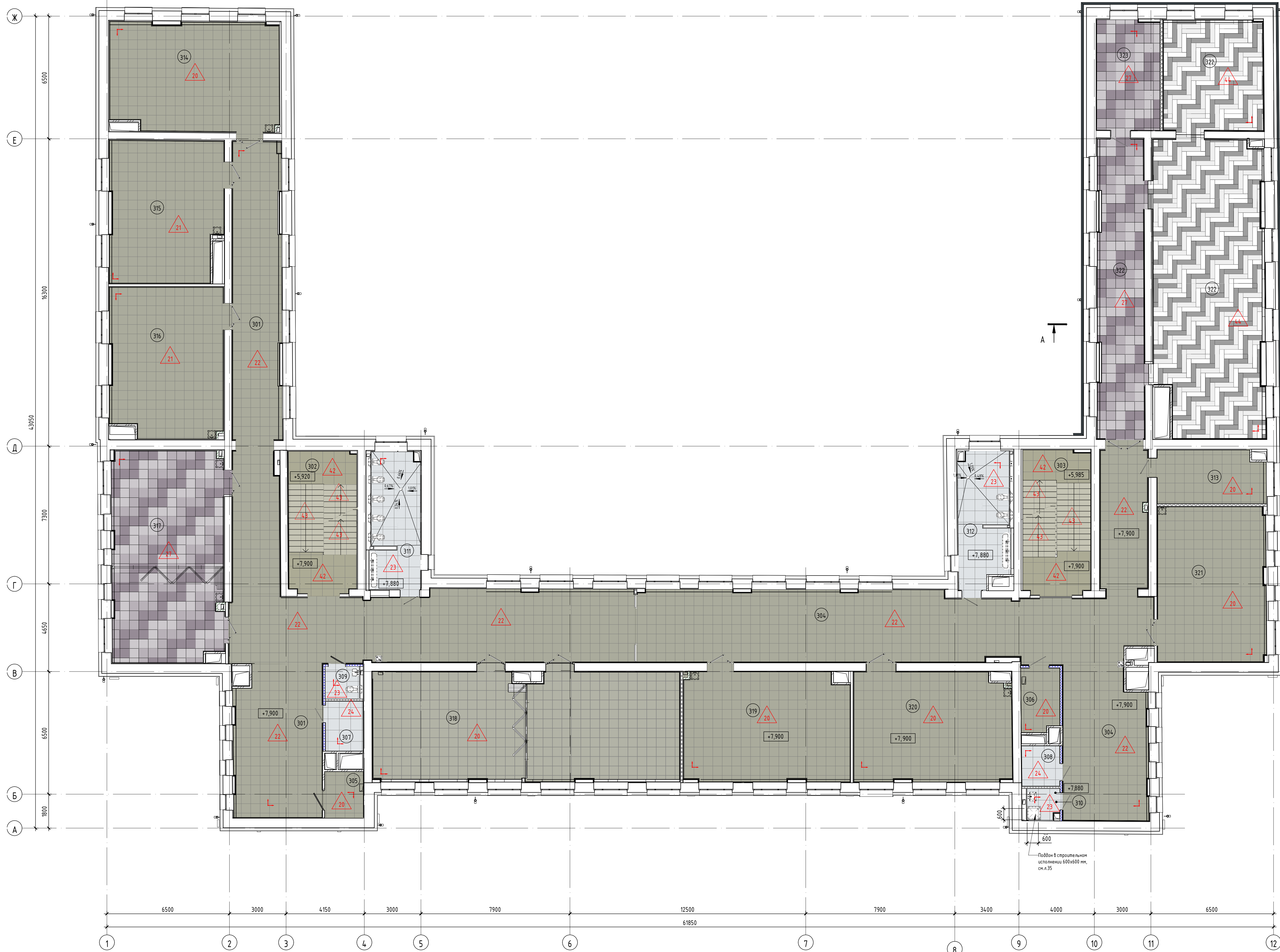
План полов 3-го этажа
