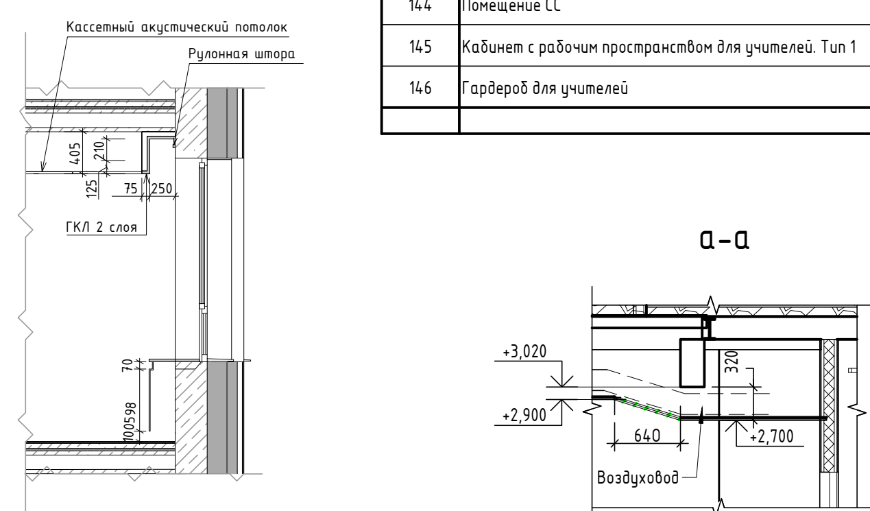
Схема устройства ниши для рулонной шторы
